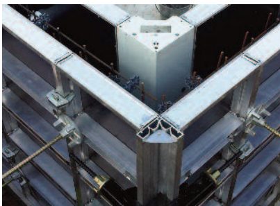
Angle ALU EXTÉRIEUR assemblé
