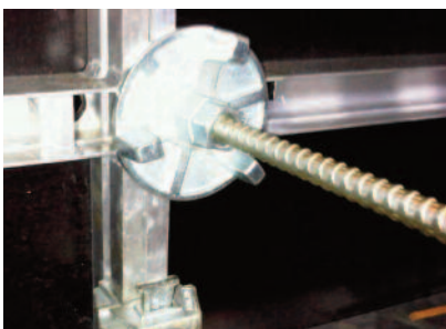
Assemblage tige écrou
